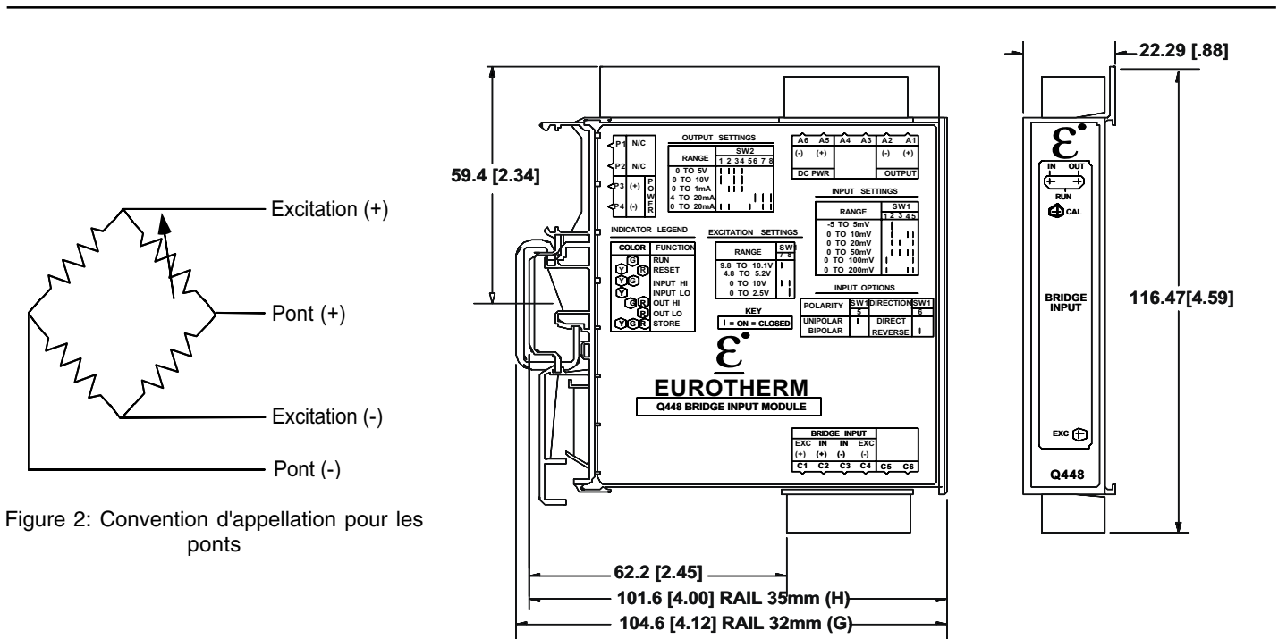
Figure 3: Dimensions mécaniques du Q448
