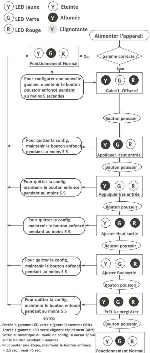
Figure 1: Procédure de calibrage
